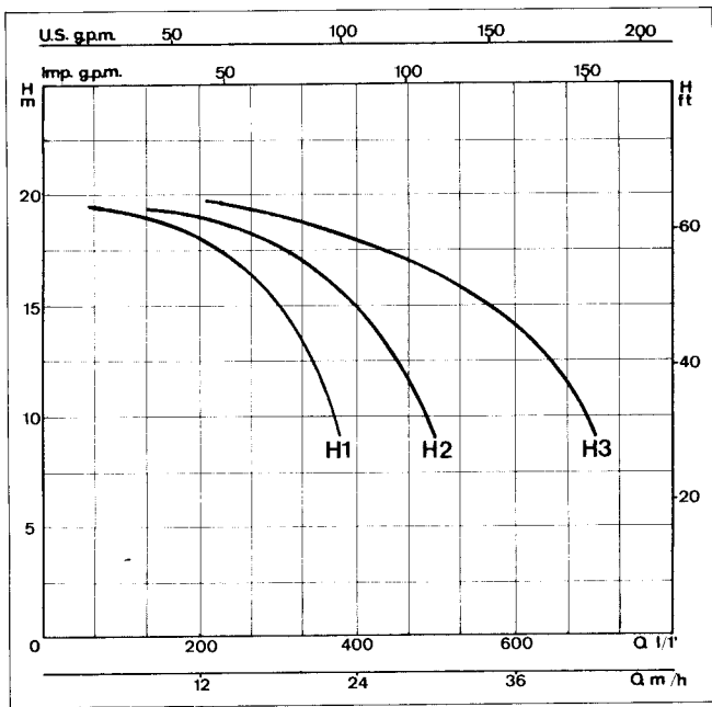
Curve di funzionamento a 3000 giri/1''
